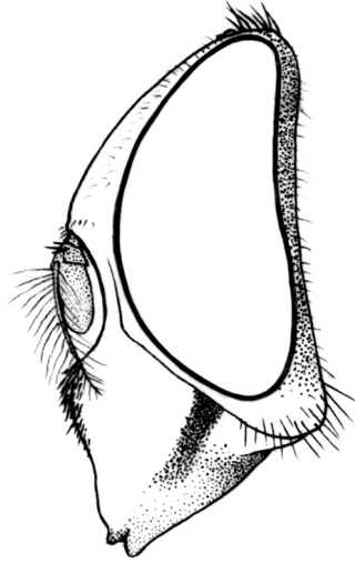
图 372 黑鬃蜂蚜蝇 Volucella inanis (Linnaeus)
